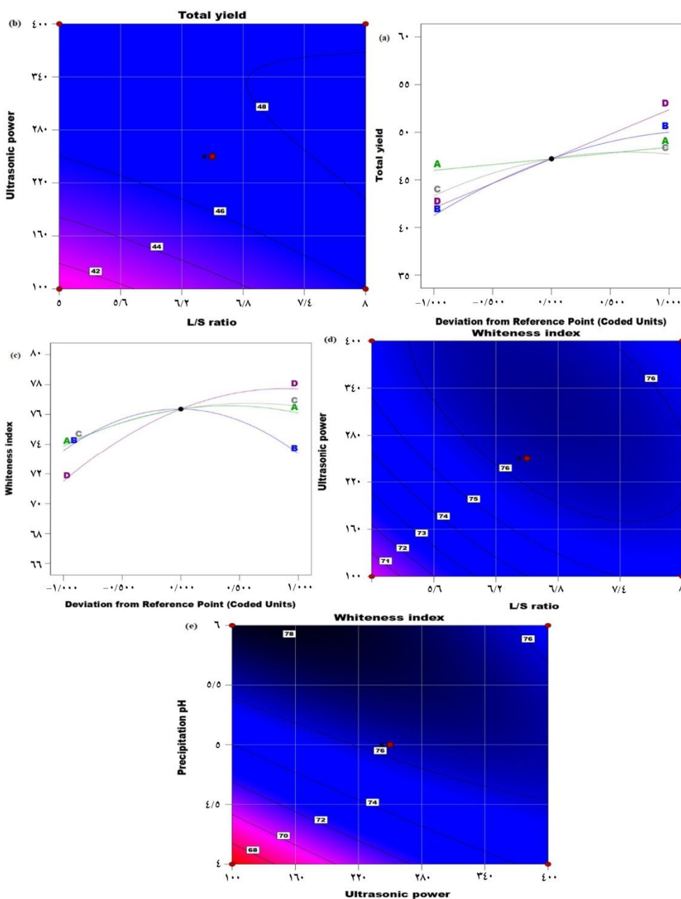
شکل ۲- نمودارهای نشان‌دهنده اثر متغیرهای مستقل به شکل تک شامل نسبت مایع به جامد (A)، pH انحلال (B)، توان دستگاه التراسونیک (C) و pH ترسیب (D) و نمودارهای کانتور رگرسورهای بهمکنش حفظ شده در مدل بر متغیرهای پاسخ درصد بازدهی کل (a و b) و شاخص سفیدی (c تا e).
