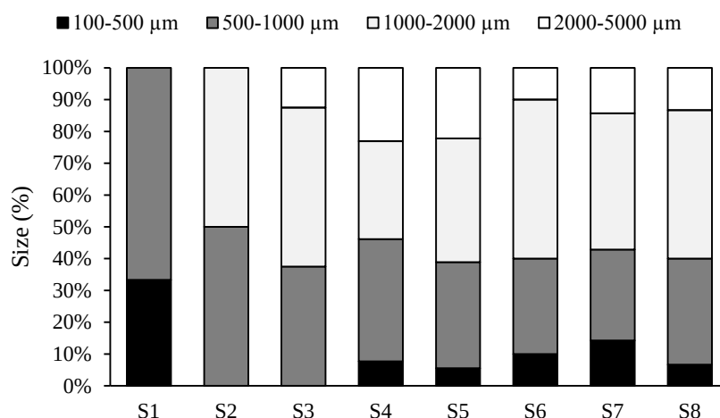
شکل ۳- درصد فراوانی اندازه‌های مختلف میکروپلاستیک‌ها در ایستگاه‌های تالاب گمیشان.
