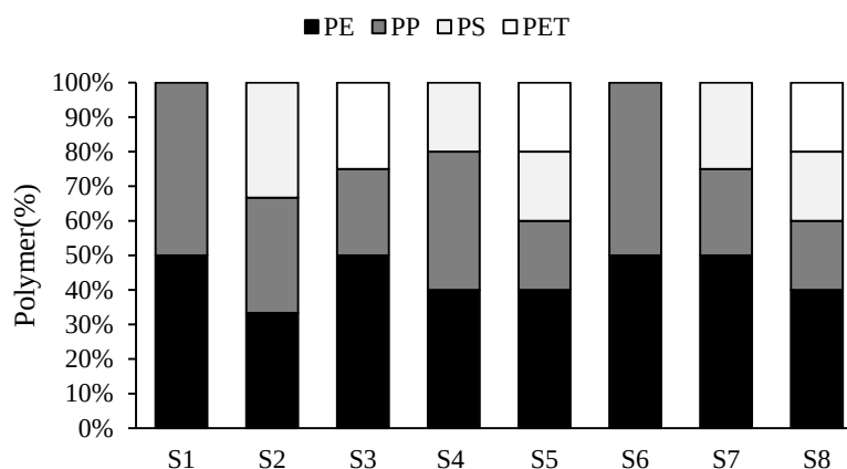
شکل ۷- درصد فراوانی انواع پلیمرهای میکروپلاستیک‌ها در ایستگاه‌های تالاب گمیشان.
