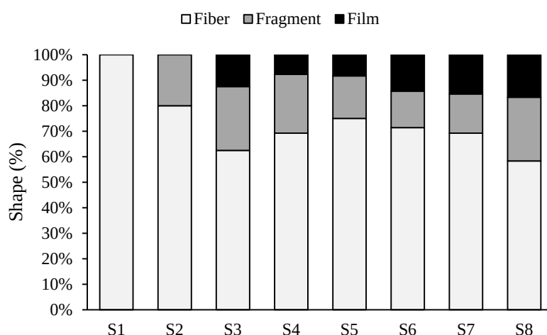
شکل ۵- درصد فراوانی شکل‌های مختلف میکروپلاستیک‌ها در ایستگاه‌های تالاب گمیشان.
