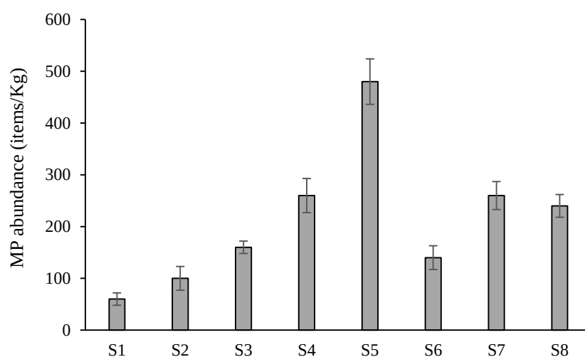
شکل ۲- درصد فراوانی میکروپلاستیک‌ها در ایستگاه‌های تالاب گمیشان.
