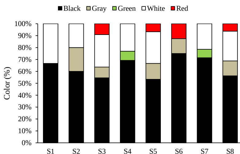
شکل ۴- درصد فراوانی رنگ‌های مختلف میکروپلاستیک‌ها در ایستگاه‌های تالاب گمیشان.
