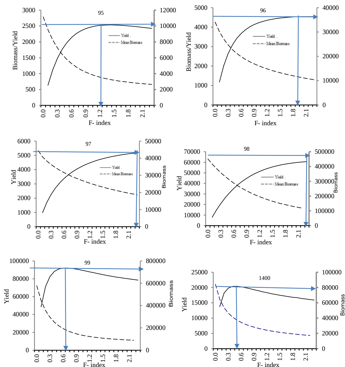
شکل ۵- نمودار تغییرات تولید (کیلوگرم) براساس ضرایب مرگ و میر صیادی ماهی کپور با استفاده از مدل تامپسون و بل در سال‌های ۱۳۹۵-۱۴۰۰.
