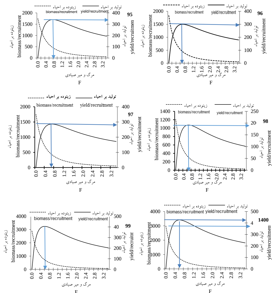
شکل ۴- منحنی تولید بر احیاء ماهی کپور در جنوب‌شرقی دریای خزر با مقادیر L_r و L_c در سال‌های ۱۳۹۵-۱۴۰۰.
