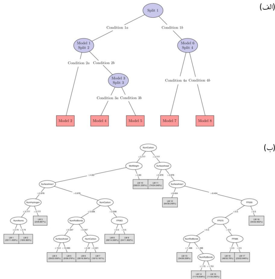
شکل ۴- نمای شماتیک یک مدل درختی رگرسیونی (الف)؛ یک مدل درخت رگرسیونی نهایی برای یک مجموعه داده (ب).
