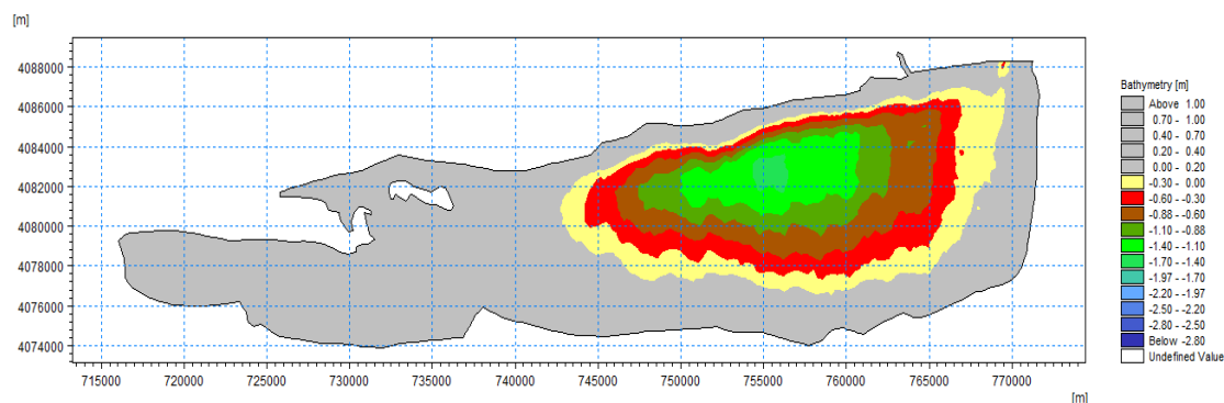
شکل ۳- هیدروگراف خلیج گرگان در سال ۱۴۱۹ خورشیدی و در سناریوی خوش‌بینانه.
