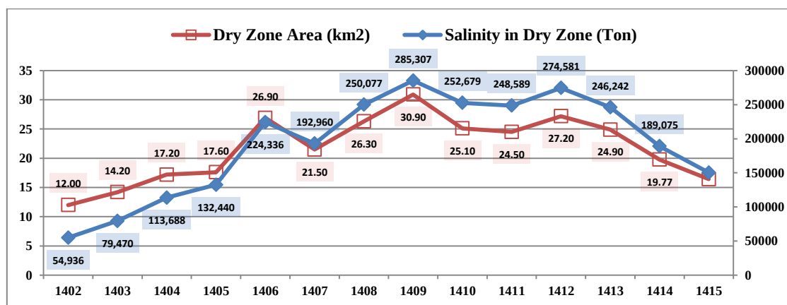
شکل ۸- منحنی میزان شوری دریافتی توسط سواحل در مقایسه با مساحت خشکی‌زائی در خلیج گرگان در سناریو بینابینی.
