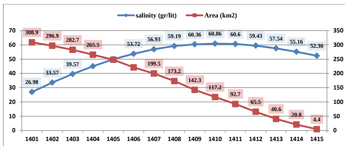
شکل ۷- منحنی تغییرات شوری خلیج در مقایسه با تغییرات مساحت خلیج گرگان در سناریو بینابینی.
