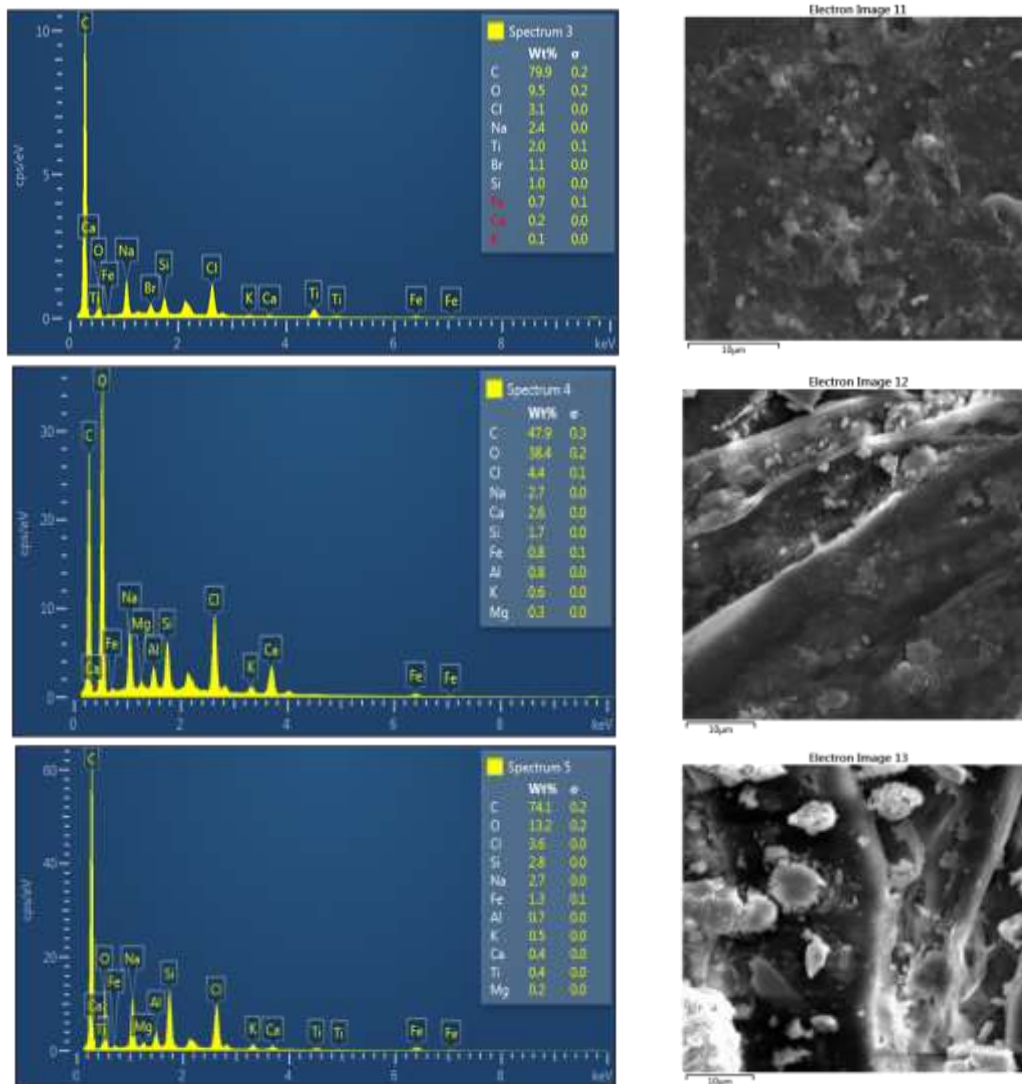
شکل ۵- آنالیز FESEM-EDS مربوط به سه نمونه میکروپلاستیک.
